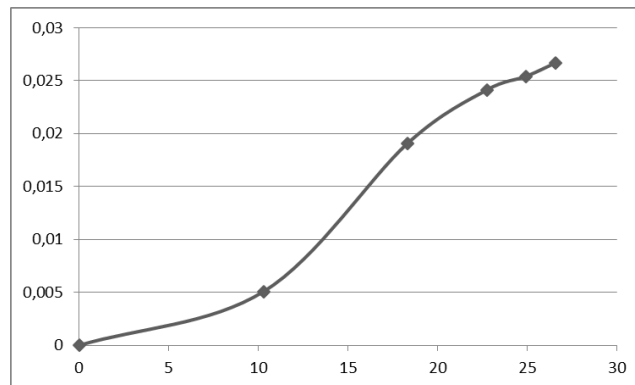
Рис. 1 Визначення поглинальної здатності піщаного ґрунту по іону купрум(II)
