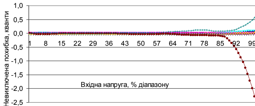
Рис. 2 Залежність невиключеної похибки нелінійності АЦП від вхідної напруги для відхилення
