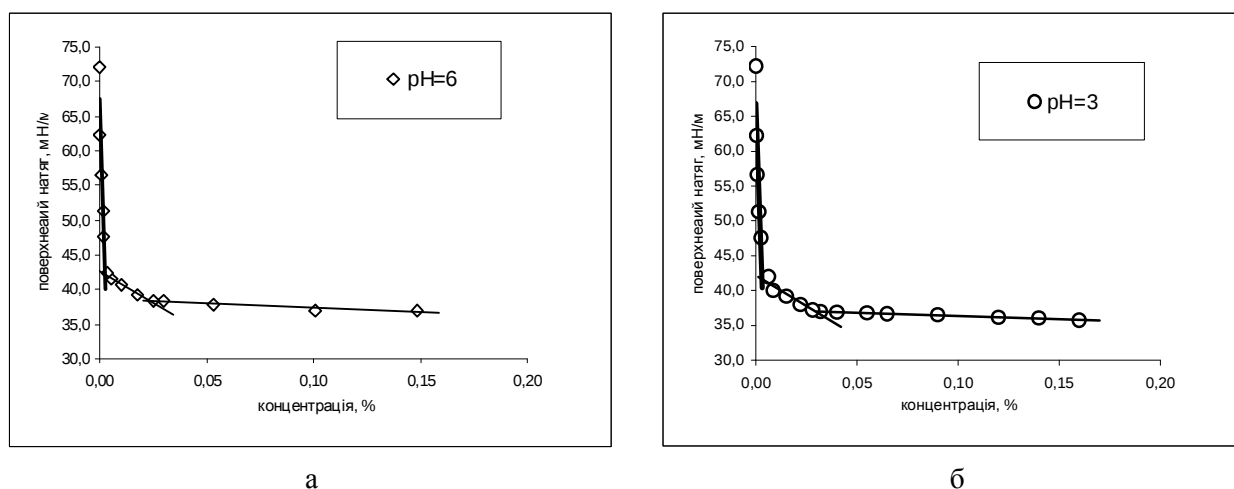
Рис. 5. Ізотерми поверхневого натягу для амфіфільного поліестерету ко-(GluSt-DPG-GluSt)-ко-PEG1000 визначенні за різних pH-середовищ: а – за pH=6; б – за pH=3
