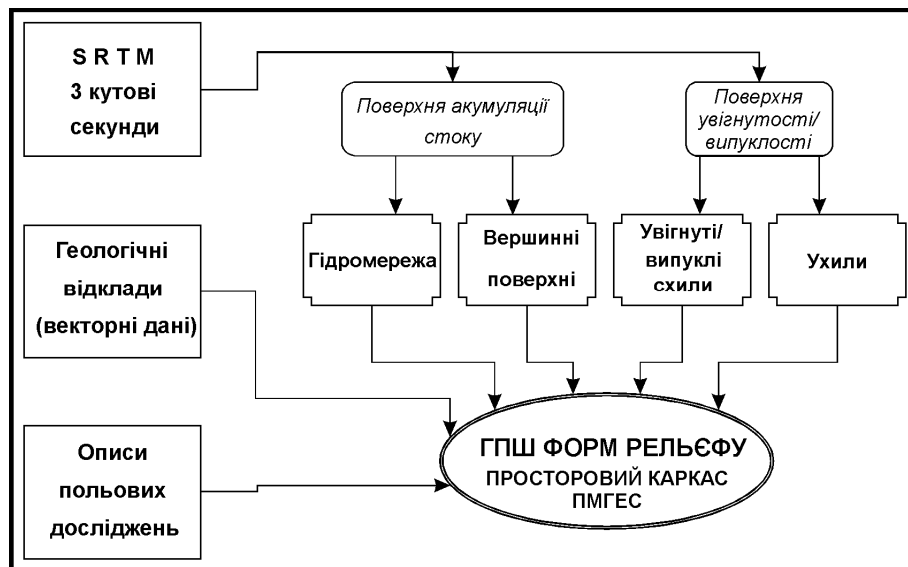
Рис. 3. Схема напівавтоматизованої делімітації просторового каркасу природних морфогенних геоєкосистем
