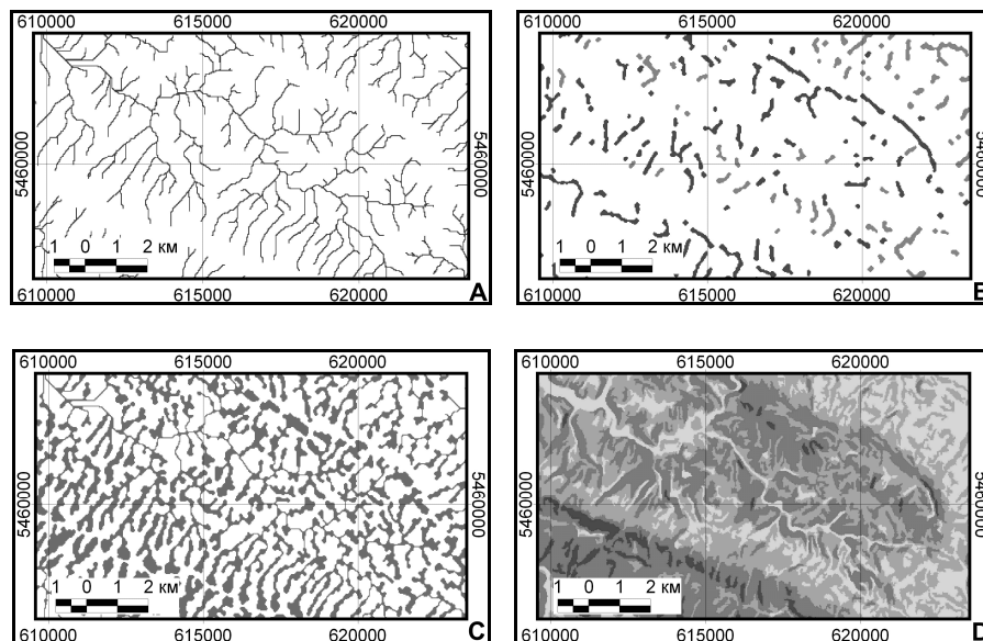
Рис. 4. Фрагменти тематичних ГПШ на ділянці між хребтами Отрит та Остре
