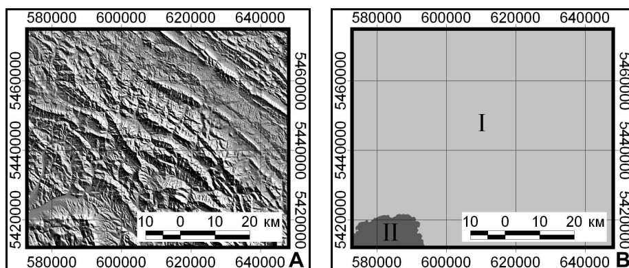
Рис. 2. Цифрова модель рельєфу (А) та геологічні відклади (В)
