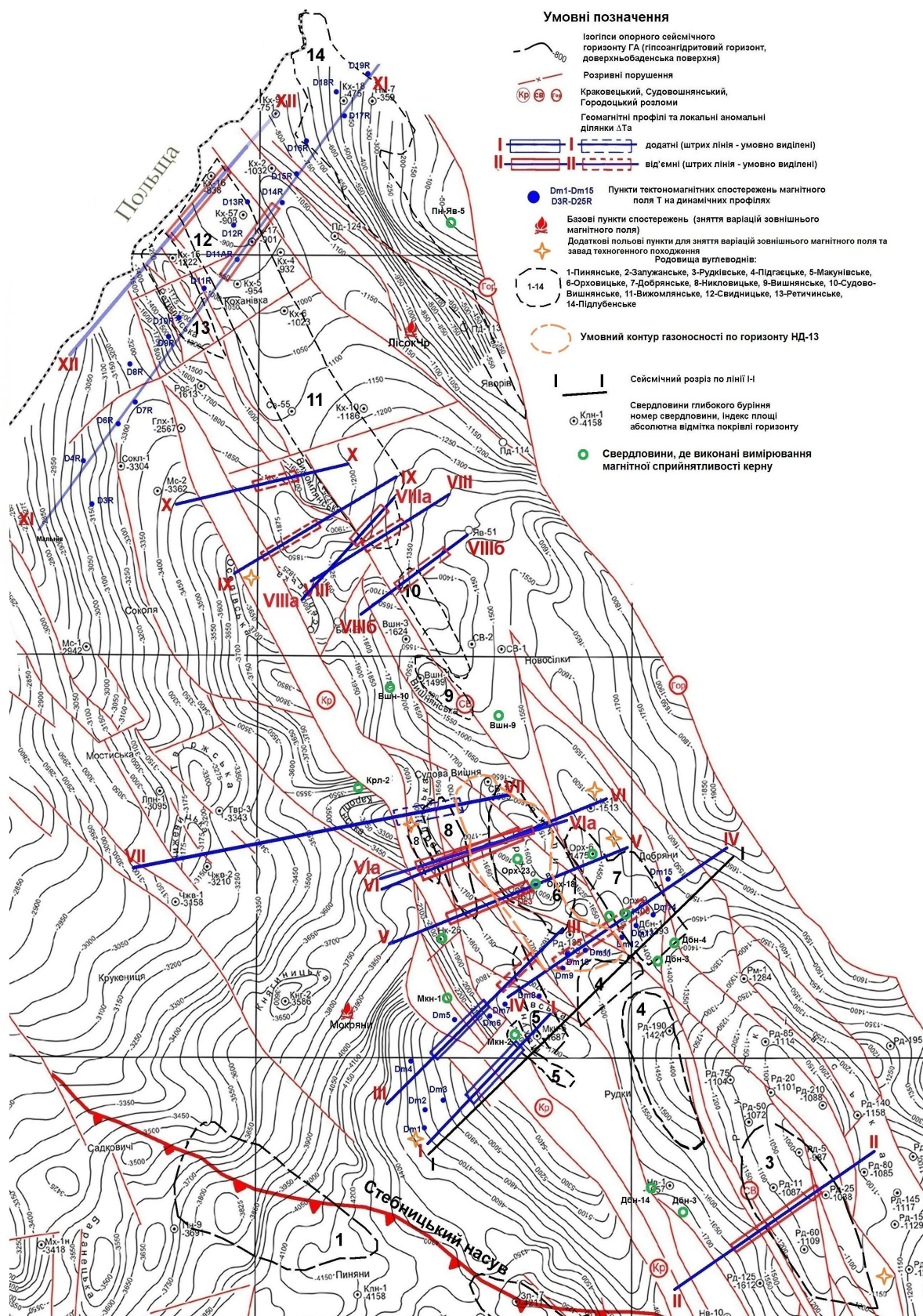
Рис. 2. Структурна карта гіпсоангідритового горизонту (за матеріалами ЗУГРЕ) та геомангнітні профілі із локальними аномальними ділянками \Delta F_a Fig. 2. Structural map of gypsum-anhydrite layer (the seismic data from “Ukrgeofizyka” West Ukrainian Geophysical Prospecting Expedition) and geomagnetic profiles with the section of local magnetic anomalies \Delta F_a
