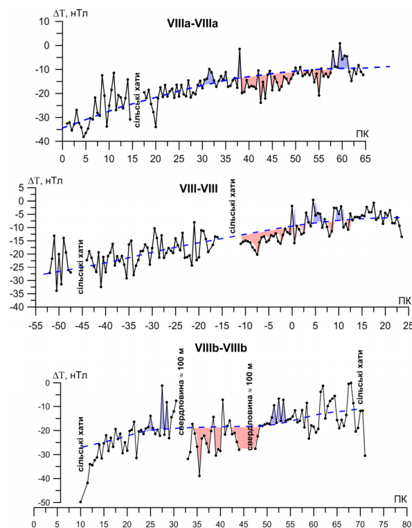
Рис.4. Різницеve магнітне поле \Delta T та локальні магнітні аномалії \Delta T_a на Вижомлянській і Судово-Вишнянській структурах (ум. позначення на рис. 3)
