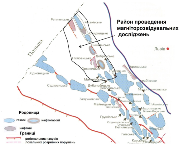
Рис. 1. Схема розташування нафтогазових родовищ у північно-західній частині Більче-Волицької зони Передкарпатського прогину Fig. 1. Location of oil and gas fields in the NW part of Bilche-Volytsa zone in Carpathian Foredeep
