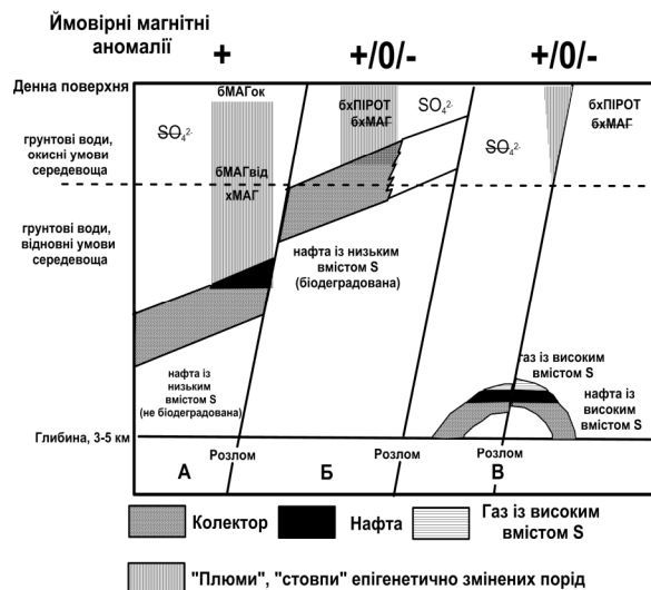
Рис. 7. Схематичні моделі пасток вуглеводнів та ефект у магнітному полі від мінералогічних змін порід під впливом мікропросочування флюїдів вуглеводнів (бМАГ ок – утвор. за участі бактерій в окисних умовах, бхПІРОТ – бакт. або хіміч. утворений піротин, бМАГ від – магнетит бакт. у відновних умовах, бхМАГ – бакт. або хіміч. утворений магнетит, хМАГ – хімічно утворений магнетит), [Machel H.G., 1991b]
