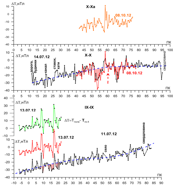
Рис. 5. Різницеве магнітне поле \Delta T та локальні магнітні аномалії \Delta T_a на Вижомлянській структурі Fig. 5. Difference \Delta F magnetic field and local magnetic anomalies \Delta F_a on the Vigomlia structure
