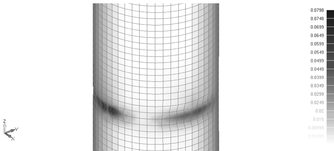
Рис. 8. Схема деформування та розподілу поверхневих напружень бетонного ядра труботетонної колони вузла із зовнішніми ребрами
