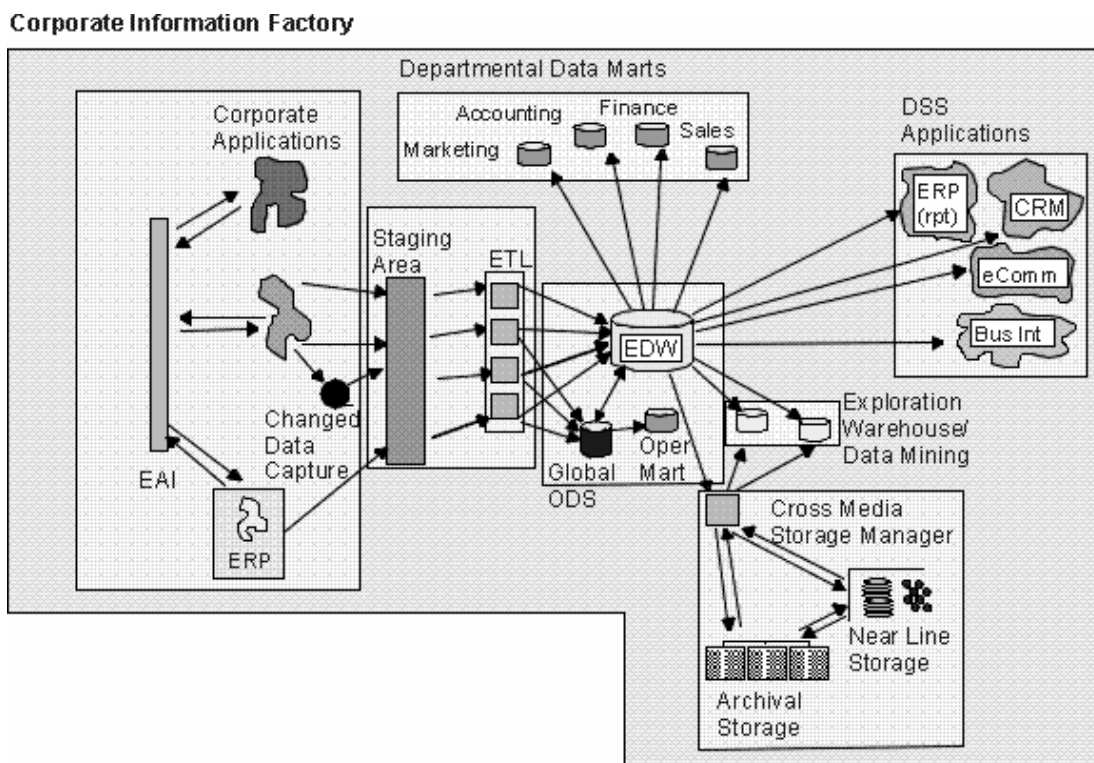
Рис. 2. Архітектура корпоративної інформаційної фабрики [4]
