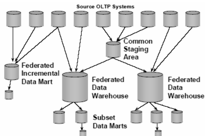
Рис. 3. Архітектура об'єданого сховища даних
