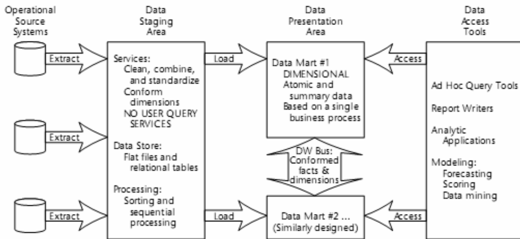
Рис. 1. Архітектура багатовимірного сховища даних
