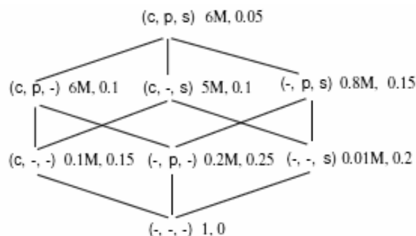
Рис. 4. Решітка кубів
