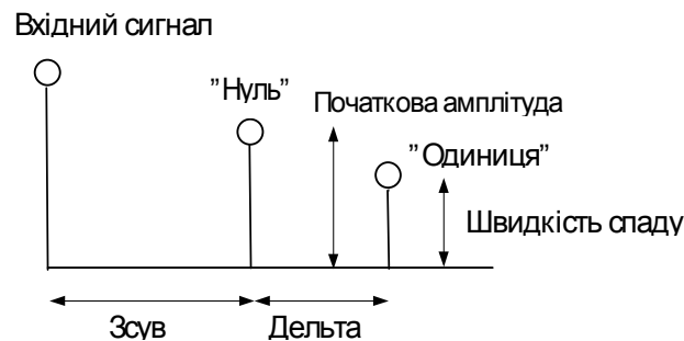
Рис. 2. Параметри ехо-сигналу
