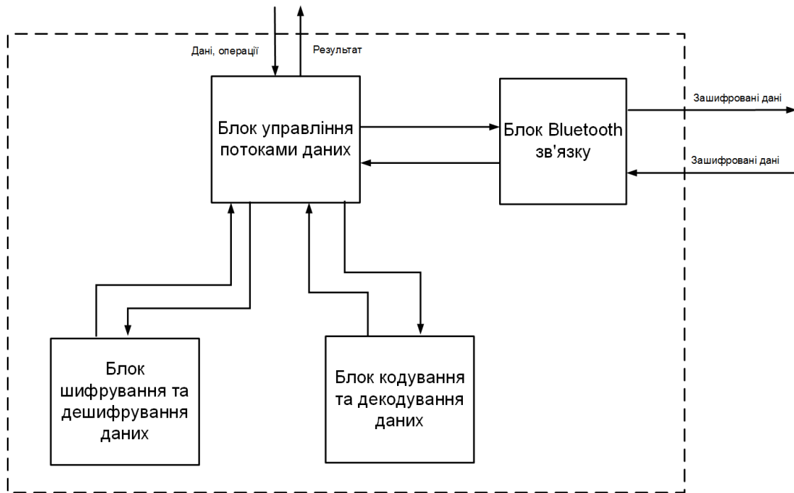
Рис. 2. Структурна схема системи криптографічного захисту Bluetooth зв'язку між пристроєм інтернету речей та мобільним обчислювальним пристроєм
