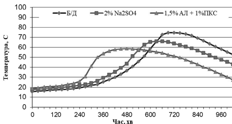
Рис. 3. Вплив лужних прискорювачів на кінетику зміни температури гідратації композиційного портландцементу ПЦ ІІ/Б-К-400Р-Н
