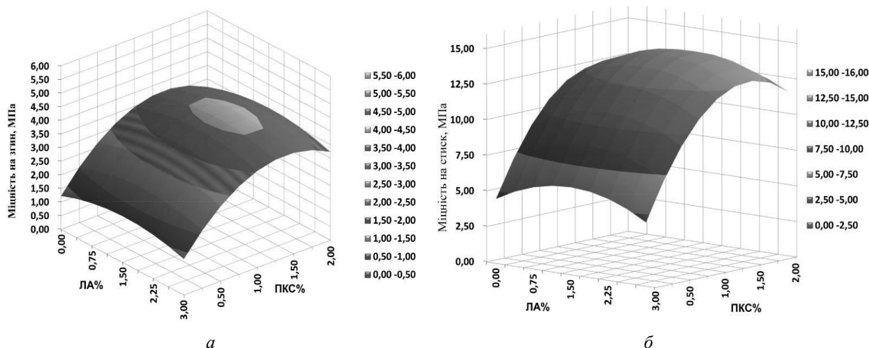
Рис. 2. Поверхні відгуку зміни границі міцності на згин (а) та стиск (б) дрібнозернистого бетону через 1 добу
