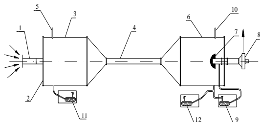
Рис. 1. Схема експериментальної установки. (10, п/ц, курсив)
