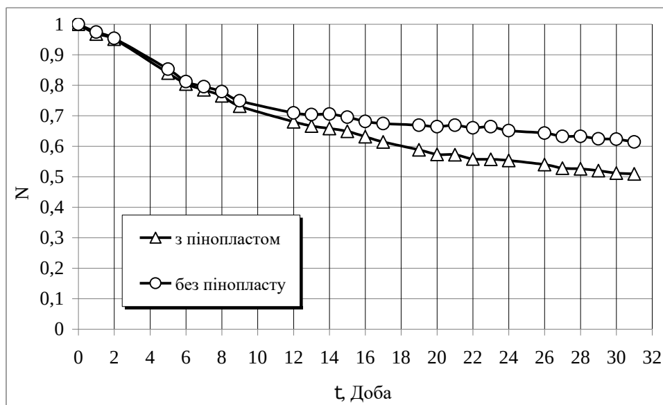
Рис. 4. Кінетика зміни відносної концентрації амонійного азоту в інфільтраті від добавки в систему носіїв для іммобілізації біоценозу.
