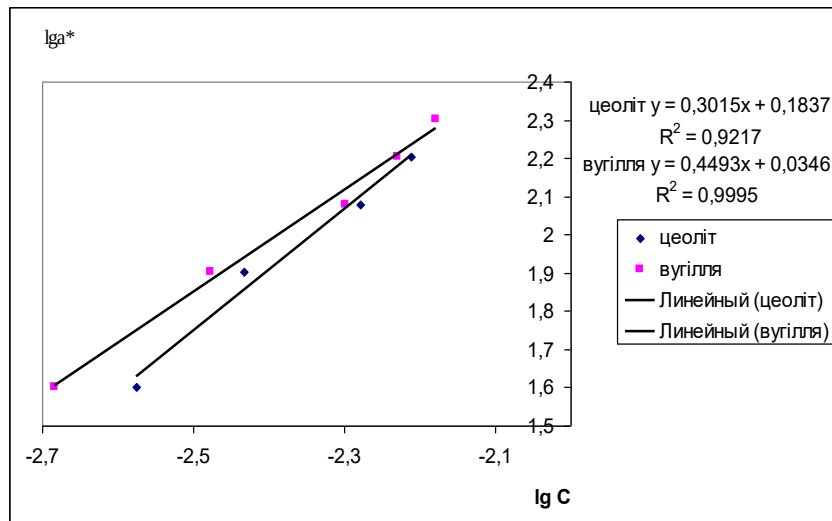
Рис. 3. Ізотерма адсорбції \alpha -оксіпропіонової кислоти на цеоліті та активованому вугіллі за Фрейндліхом в лінійних координатах
