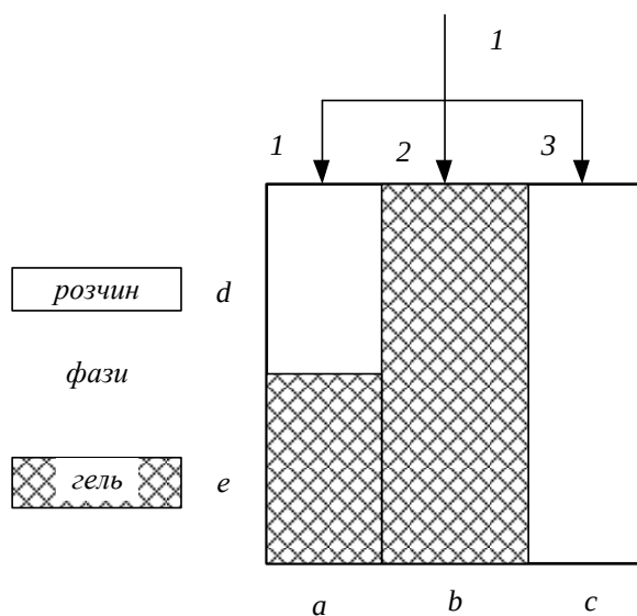
Рис. 6. Схематичне зображення трьохпровідної моделі провідності іонообмінника
