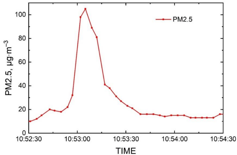
Рис. 11. Вимірювання концентрації PM2.5 при проїзді трактора на відстані 1.5 м від нерухомого приладу
