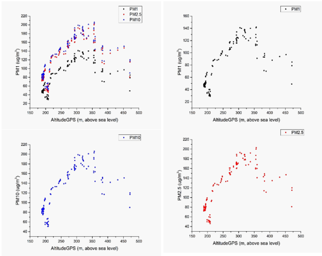
Рис. 15. Залежність концентрацій РМ1, РМ2.5, РМ10 від висоти над рівнем моря за вимірюваннями з розробленим приладом, встановленим на квадрокоптері.
