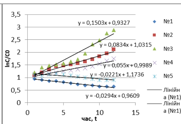
Рис. 4. Залежність зміни логарифму концентрації клітин в суспензії мікрободоростей від часу (за відповідних значень концентрацій активатора \text{H}_2\text{PO}_4^- та постійної інгібітора \text{HSO}_3^- )
