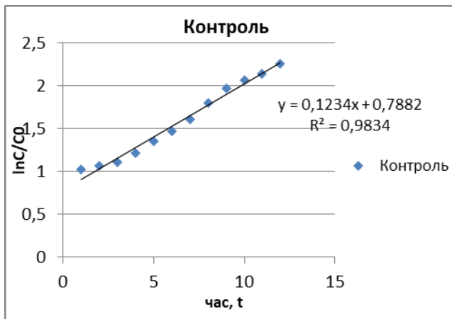
Рис. 5. Залежність зміни логарифму концентрації клітин в суспензії мікроводоростей від часу (контроль)
