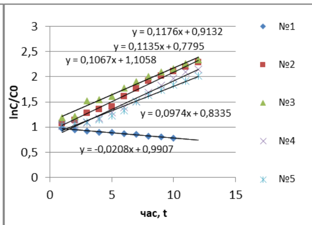
Рис. 6. Залежність зміни логарифму концентрації клітин в суспензії мікроводоростей від часу (за відповідних значень концентрацій активатора \text{NO}_3^- та постійної інгібітора \text{HSO}_3^- )
