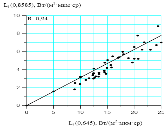
Рис. 3. Залежність мінімальних значень яскравості висхідного випромінювання, характерних для вод з мінімальними концентраціями суспензії ( L_A(8585) = 0,31[L_A(645)] , R^2 = 0,88 )
