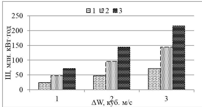
Рис. 6. Залежність зменшення електровиробництва (І) від скорочення забору води з річки ( \Delta W ): 1 – тривалість обмеження 1 доба, не працює один блок; 2 – тривалість обмеження 2 доби, на працює 2 блока; 3 – тривалість обмеження 3 доби, зупинка АЕС
