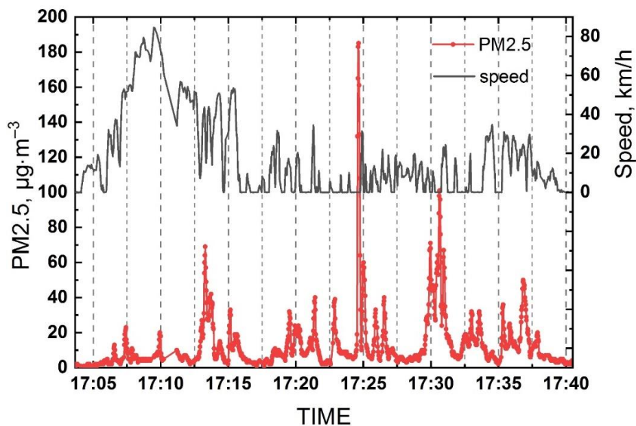
Рис. 13. Концентрація PM_{2.5} на під'їзді до Львова зі сторони Брюховичів – відрізок часу 17:05–17:16 та на вулицях Львова – відрізок часу 17:16–17:41. Вісь абсцис для графіка швидкості руху автомобіля зміщена вгору.
