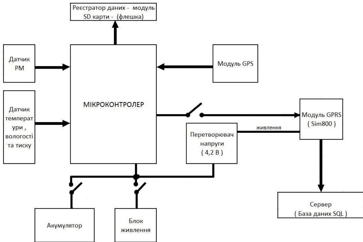
Рис. 2. Блок-схема запропонованого приладу реєстрації концентрації аерозолію
