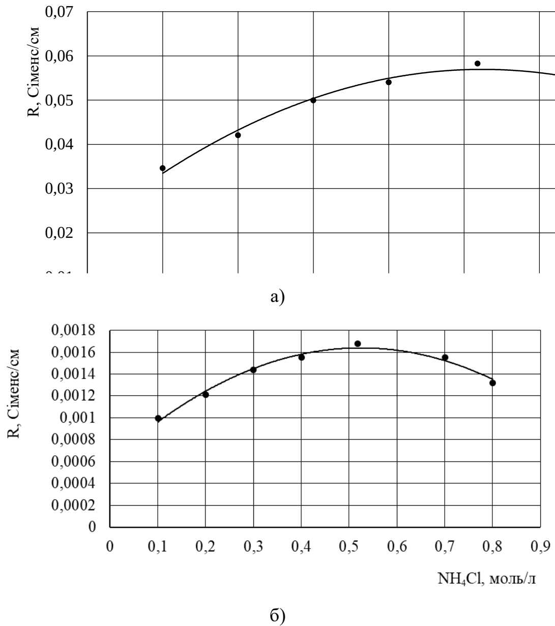
Рис.2. Опір системи іоніт-розчини \text{NH}_4\text{Cl} в U-подібній трубці:
