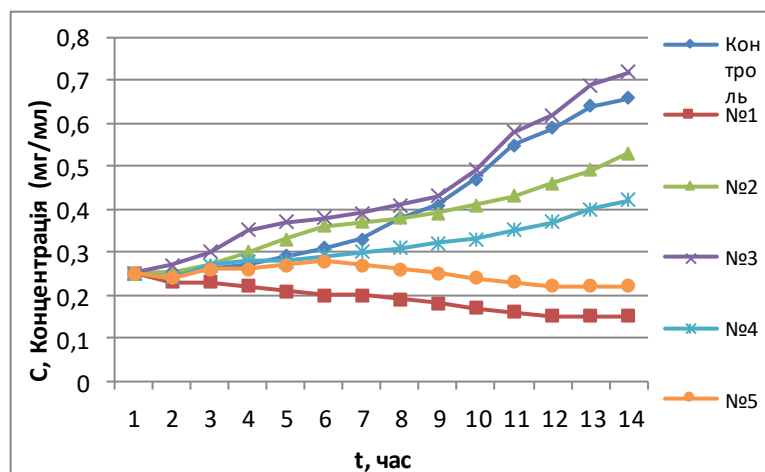
Рис. 1. Залежність зміни концентрації клітин мікроводоростей в часі за відповідних концентрацій аніону \text{HSO}_3^- та аніону \text{H}_2\text{PO}_4^-
