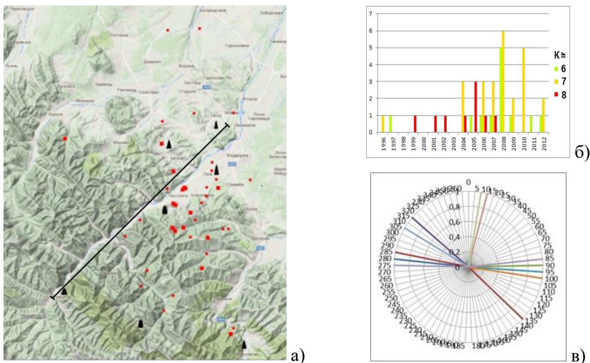
Рис. 6. Сейсмічність району Надвірної: а) – просторова локалізація вогнищ землетрусів (червоні квадратики – епіцентри подій різної магнітуди, чорна лінія – профіль Бистриця – Гвізд) на фоні рельєфу (на картооснові Google maps); б) – загальна кількість сейсмічних подій різного класу/магнітуди у районі по роках; в) – азимути простягання розривів у вогнищах сильніших з місцевих землетрусів.
