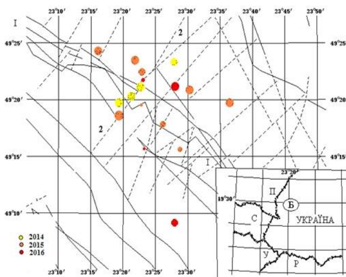
Рис. 8. Сейсмічність Бориславської зони: а) – просторова локалізація вогнищ землетрусів (кружки – епіцентри подій різної магнітуди, кольором відзначено рік події) на фоні разломної тектоніки (за В.В. Глушком та С.С. Кругловим (Глушко, Круглов, 1986) (тут: I-I – Передкарпатський розлом; 2-2 – Раточинський розлом), на врізці – локалізація Бориславської зони (Б) на оглядовій карті заходу України; б) – загальна кількість сейсмічних подій у районі по роках.
