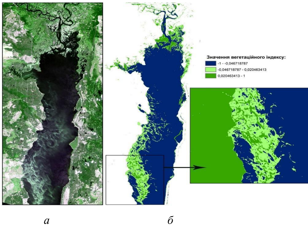
Рис. 6. Дослідження просторового розподілу ділянок цвітіння синьо-зелених водоростей на території Київського водосховища
