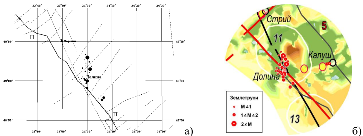
Рис. 4. Сейсмічність району Долини: а) – карта-схема просторової локалізації вогнищ землетрусів (чорні кружки – епіцентри подій різної магнітуди) на фоні розломної тектоніки району (за В.В. Глушком та С.С. Кругловим (Глушко, Круглов, 1986), тут П-П – Передкарпатський розлом); б) – землетруси району Долини на карті голоценових рухів – піднять/опускань (фрагмент карти з (Полівцев, 2011)).
