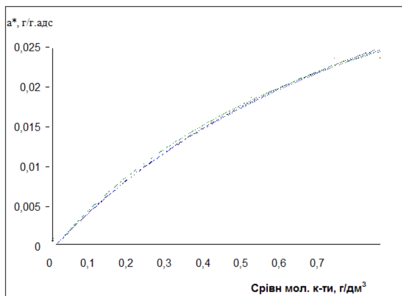
Рис. 7. Порівняння експериментальних та розрахункових даних для процесу адсорбції \alpha -оксіпропіонової кислоти на клиноптилоліті Сокириницького родовища
