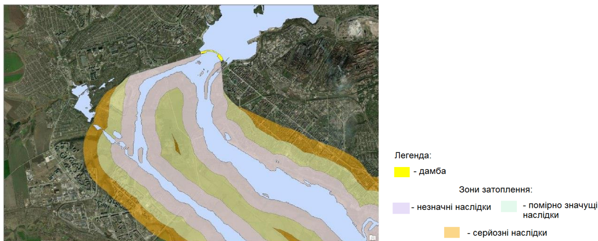
Рис. 2. 2D-модель зони затоплення Середньодніпровської ГЕС
