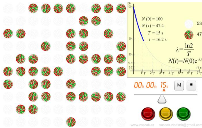
Рис. 2. Симуляція «Універсальний закон радіоактивного розпаду»
