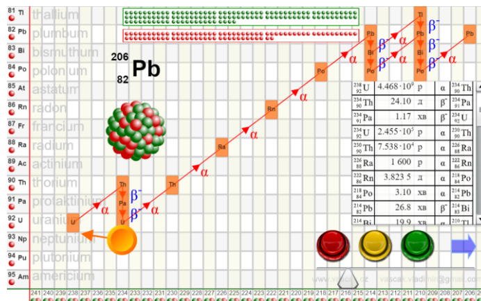
Рис. 3. Радіоактивний ряд урану U^{238}
