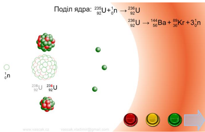
Рис. 4. Анімація «Розпад ядра \text{U}^{235} »
