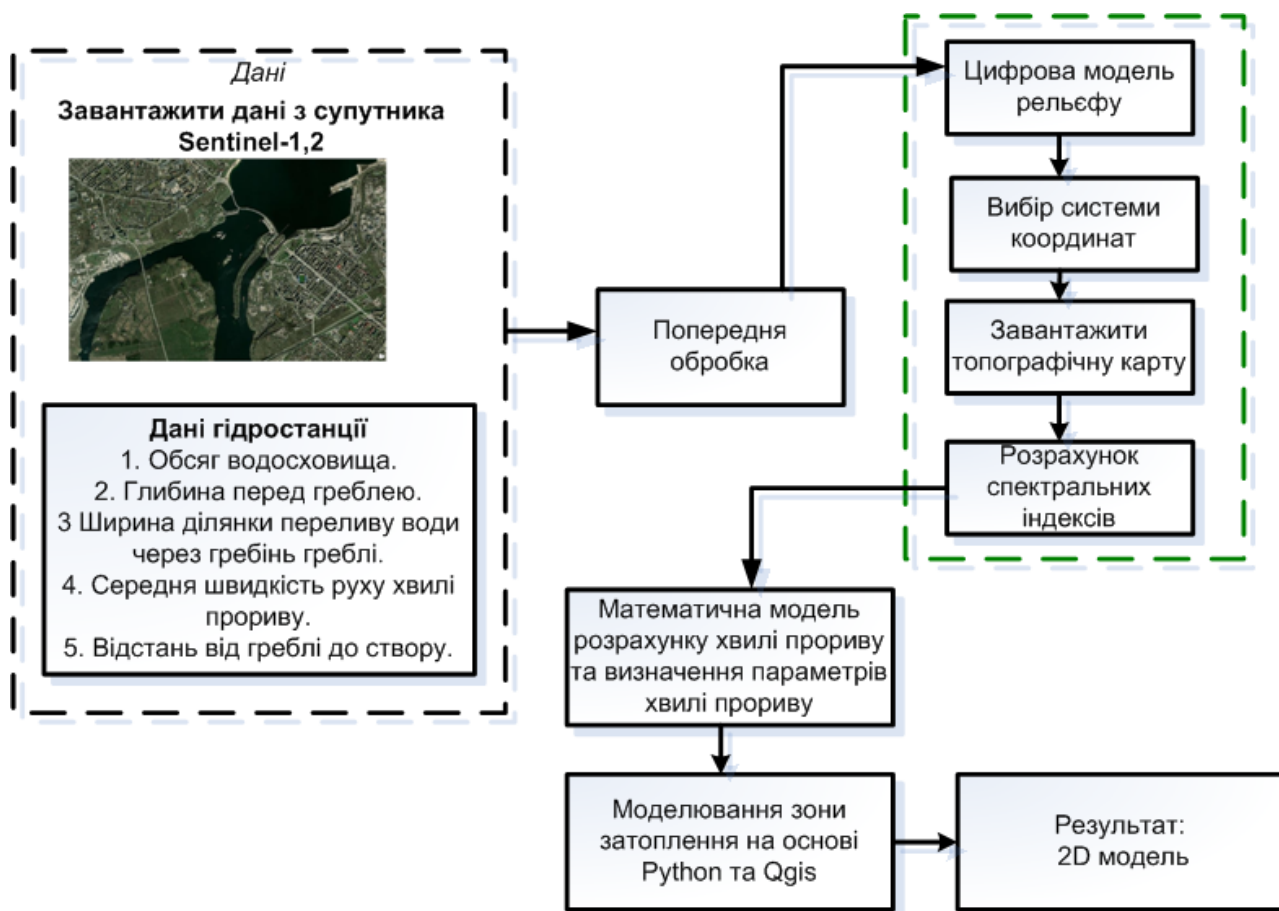
Рис. 1. Структурна схема інформаційної технології моделювання наслідків прориву гідроспоруд
