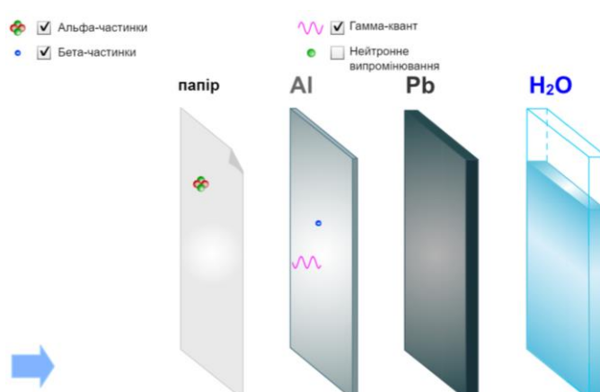
Рис. 1. Поглинання радіоактивного випромінювання різного виду речовинами
