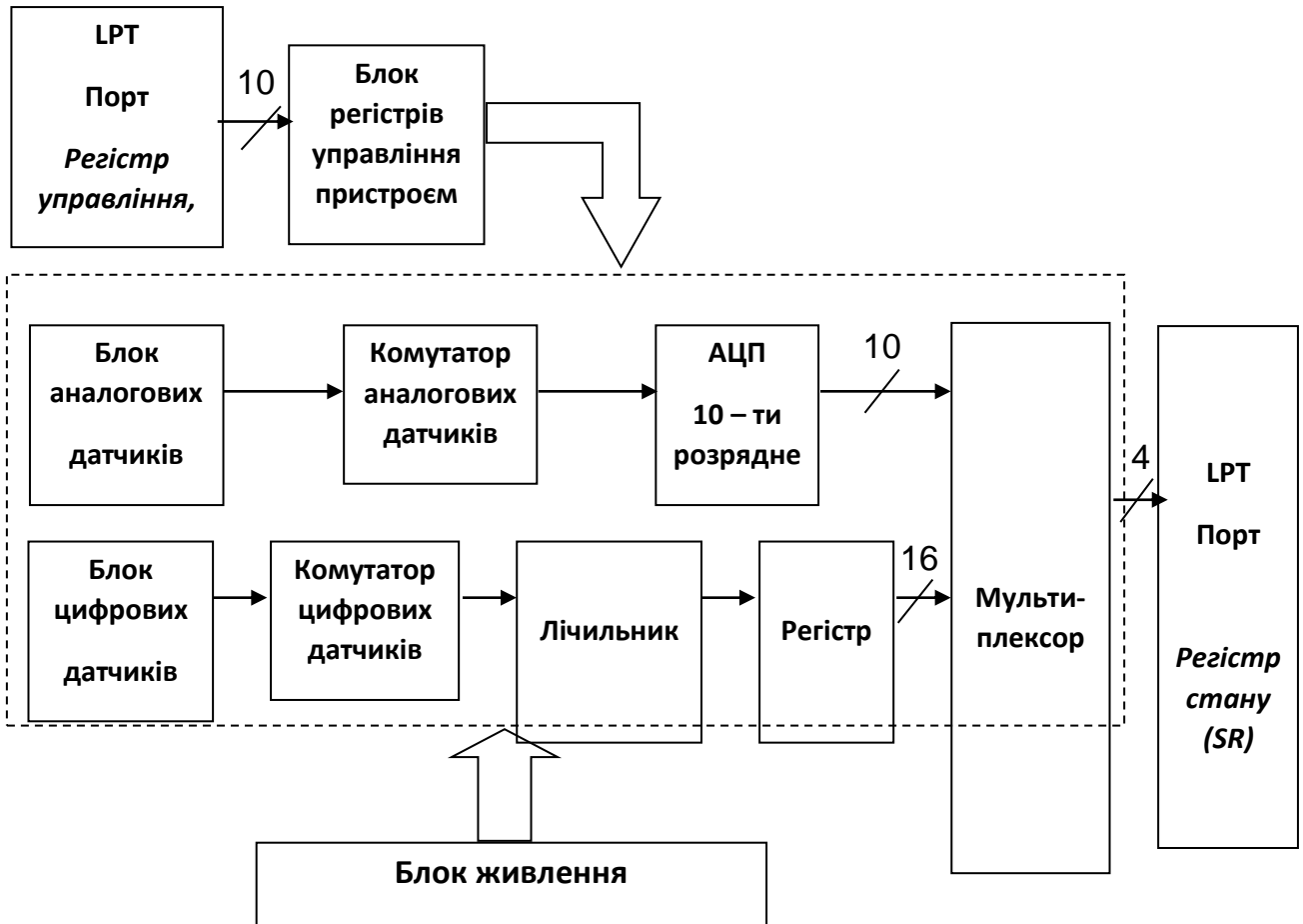
Рис. 5. Блок-схема апаратної частини комплексу
