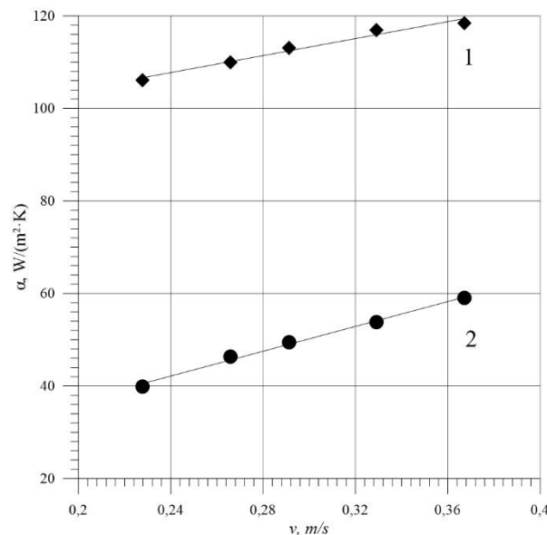
Рис. 1. Залежність коефіцієнта тепловіддачі \alpha від дійсної швидкості руху теплового агента v крізь шар: 1 – вологої сірnikової соломки, 2 – сухої сірnikової соломки.
