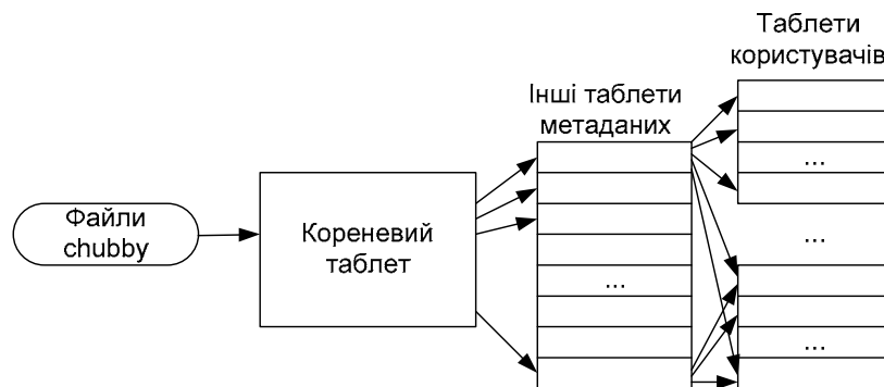
Рис. 3. Ієрархія таблетів
