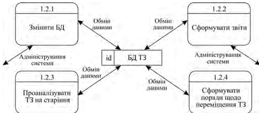
Рис. 9. DFD-діаграма системи аналізу забезпечення структурної одиниці навчального закладу третього рівня
