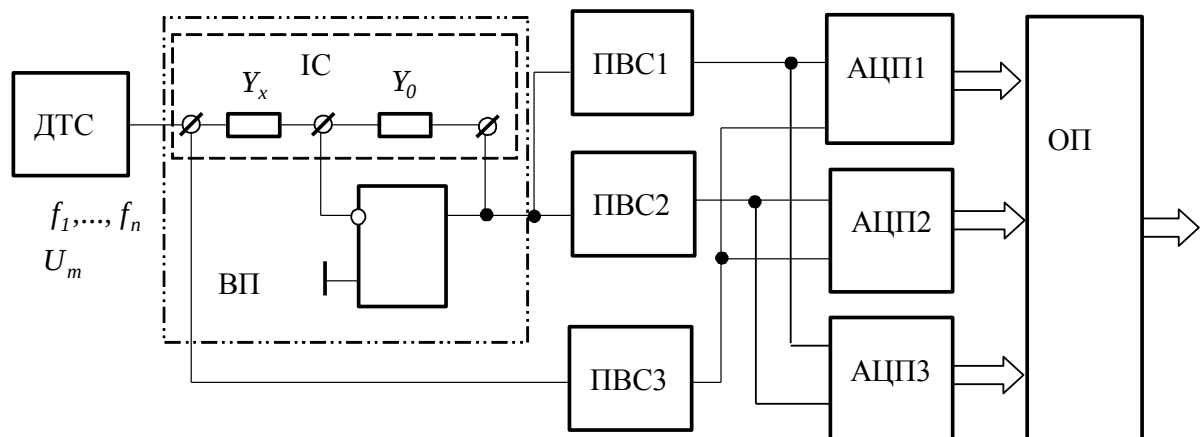
Рис.2. Структурна схема засобу з одночасним векторним перетворенням
