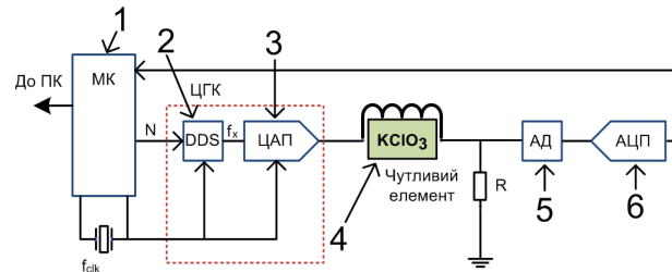
Рис. 2. Схема ЯКР на основі DDS
