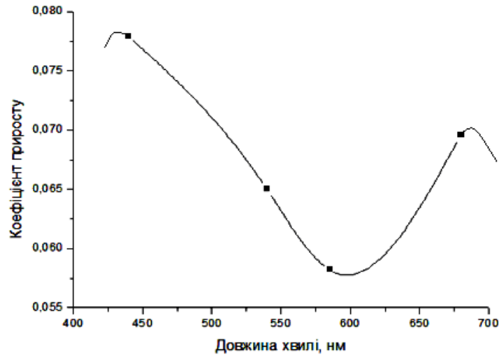
Рис. 4. Залежність коефіцієнта приросту від довжини хвилі
