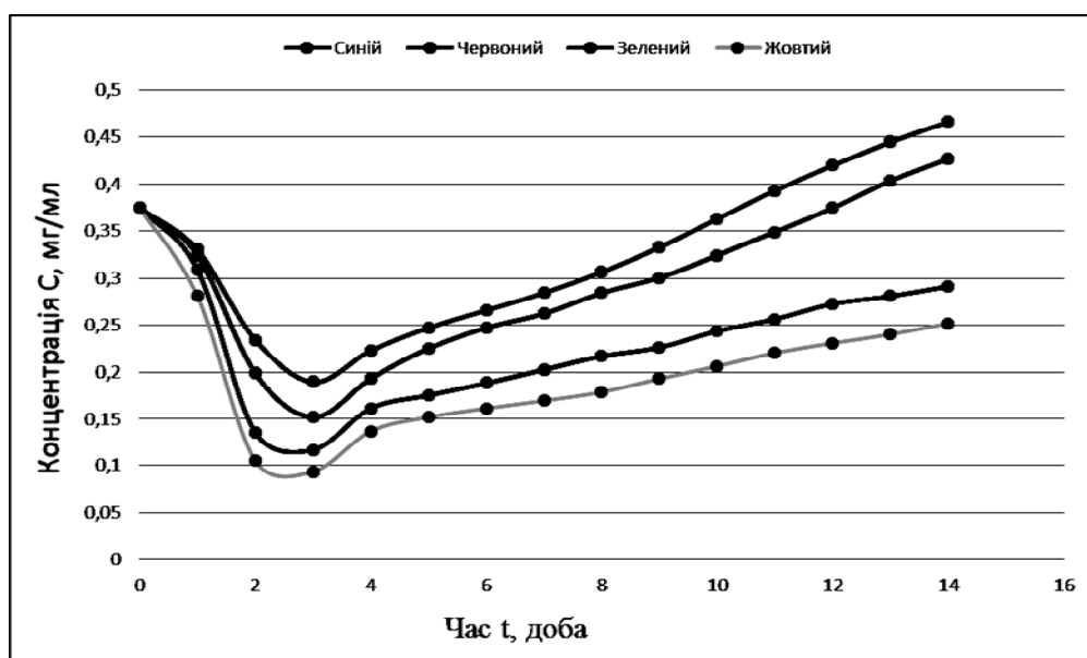
Рис. 2. Кінетичні криві приросту концентрації мікробіодоростей
