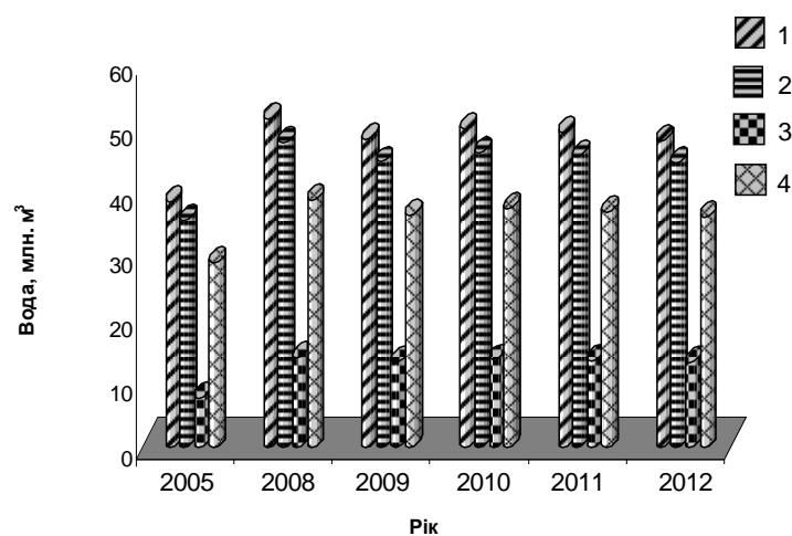
Рис. 2. Споживання та каналізування води у виробництві пива за різні роки: 1 – обсяги споживання води; 2 – кількість утворених стічних вод; 3 – кількість повністю або частково очищених стічних вод; 4 – безповоротні втрати води
