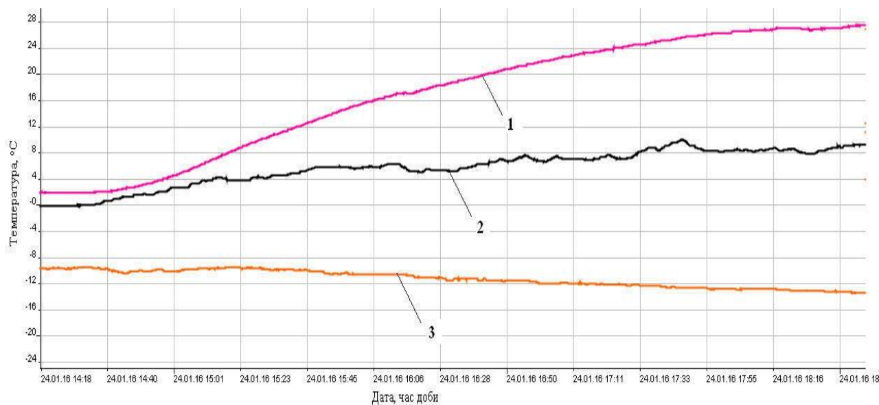
Рис. 2. Динаміка процесу нагрівання дослідного приміщення: 1 – температура поверхні покриття при підлоговому опаленні; 2 – температура повітря в приміщенні на висоті 1,5 м; 3 – температура зовнішнього повітря
