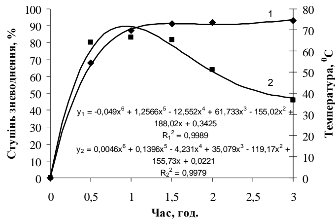
Рис. 4. Залежність ступеня зневоднення (1) та температури клиноптилоліту (2) від часу протягом оброблення в полі НВЧ-випромінювань (частота – 2,45 ГГц, потужність – 600 Вт)
