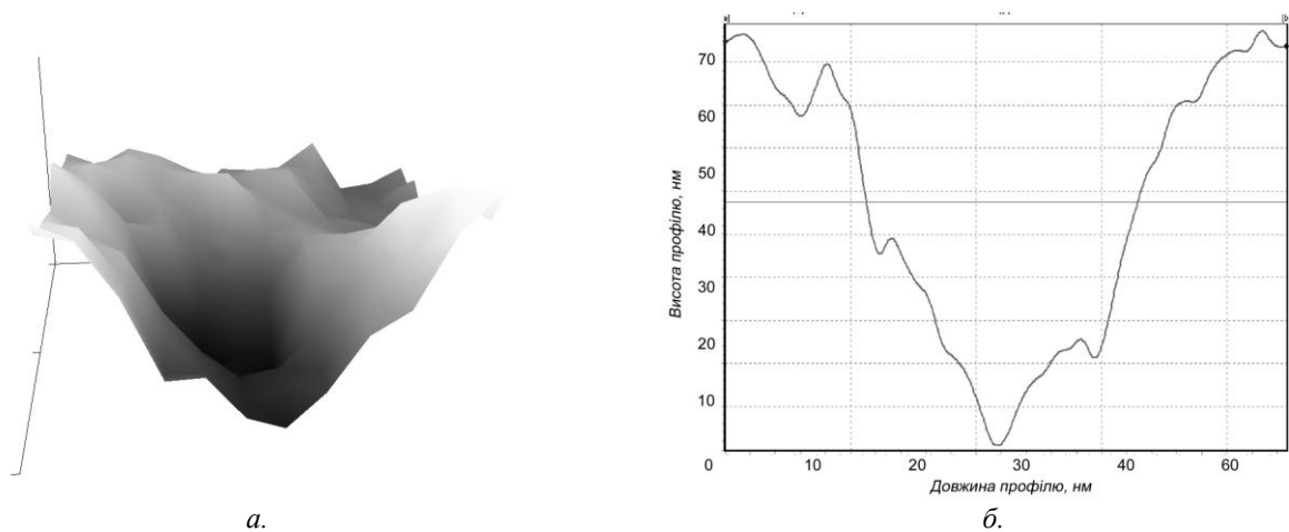
Рис. 2. Зовнішній вигляд ділянки поверхні керамічного корпусу мікрогіроскопу з відбитком наноіdentора, отриманим методом АСМ (а) та профіль відбитка АСМ-наноіdentора (б)
