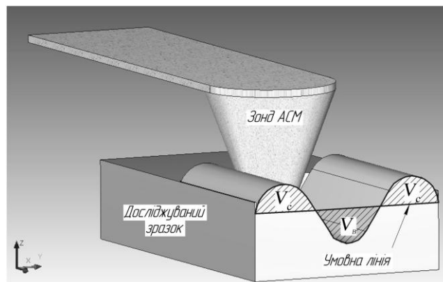
Рис. 3. Схема визначення умовного коефіцієнту зносостійкості методом склерометрії за допомогою АСМ
