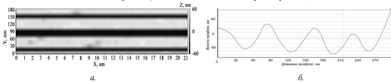
Рис. 4. АСМ-зображення (а) та топограма (б) результату склерометрії поверхні мікрогіроскопу з тонким покриттям золота (товщина 50 нм)
