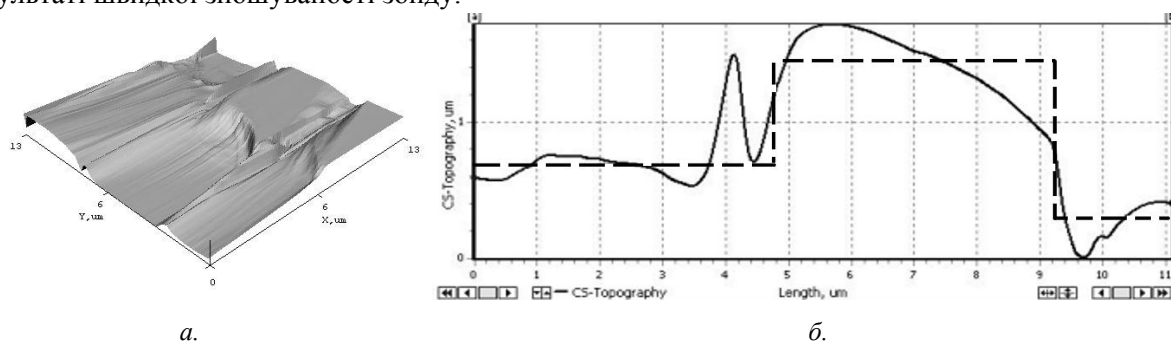
Рис. 1. Тривимірне АСМ-зображення (а) та профілограма поверхні (б) механічних наноконтактів із золота, сформованих на поверхні струмоз'ємного пристрою мікрогіроскопу.
