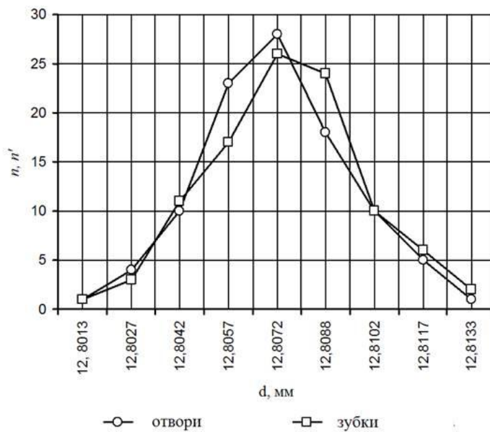
Рис. 3. Експериментальні криві суміщення розмірів отворів і зубків
