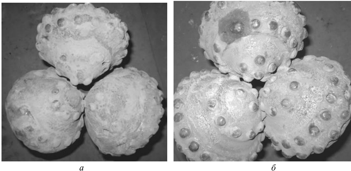
Рис. 1. Загальний вигляд зруйнованого породоруйнівного оснащення шарошок тришарошкових бурових доліт:
