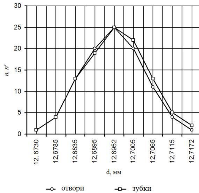
Рис. 2. Теоретичні криві суміщення розмірів отворів і зубків
