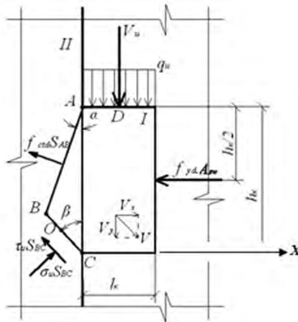
Рис. 2. Кінематично можлива схема руйнування одношпонкового стику «за шпонкою»
