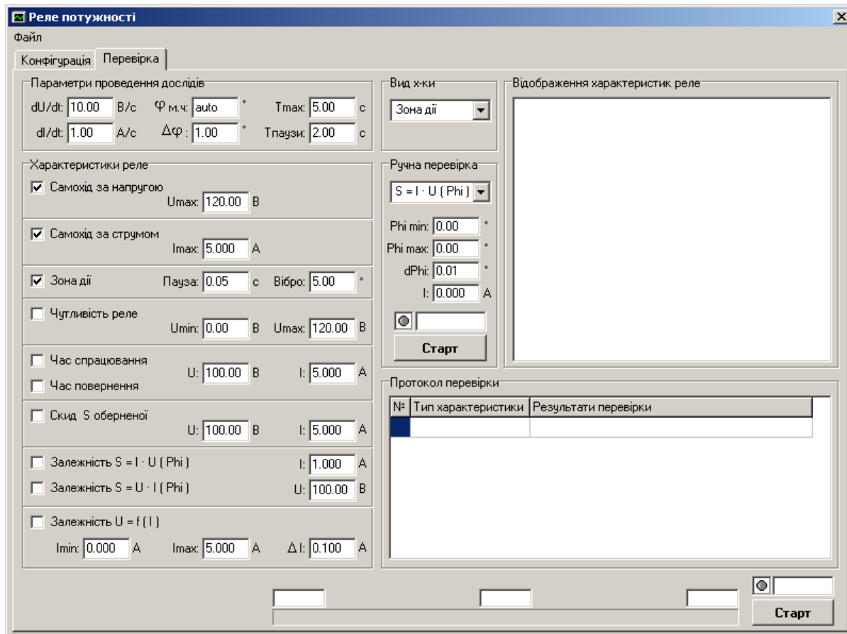
Рис. 2. Функціональна сторінка "Перевірка" реле спрямування потужності
