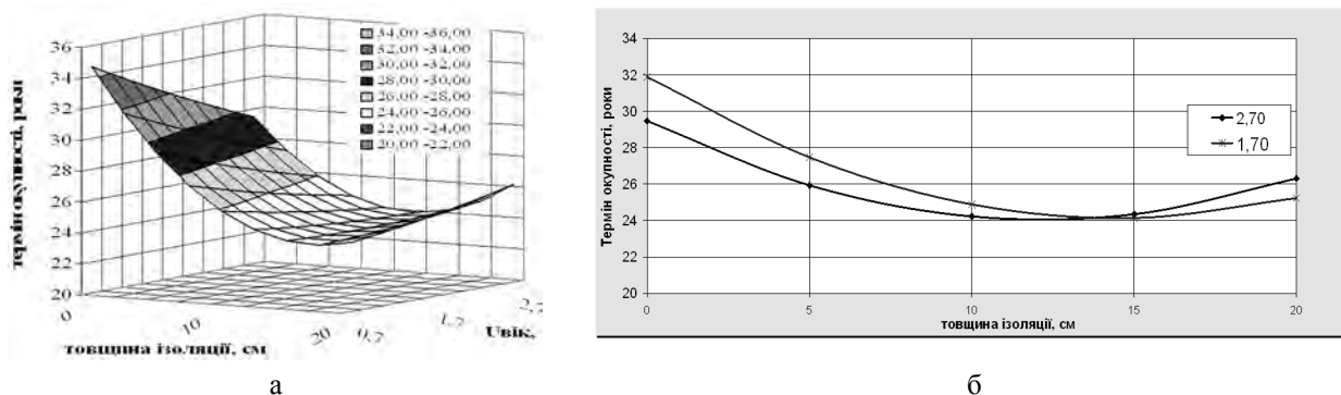
Рис. 2. Термін окупності інвестицій при реалізації варіантів проектів індивідуального будинку з механічною системою вентиляції залежно від теплотехнічних параметрів огорожувальних конструкцій (а) та від товщини теплоізоляційного шару (б)
