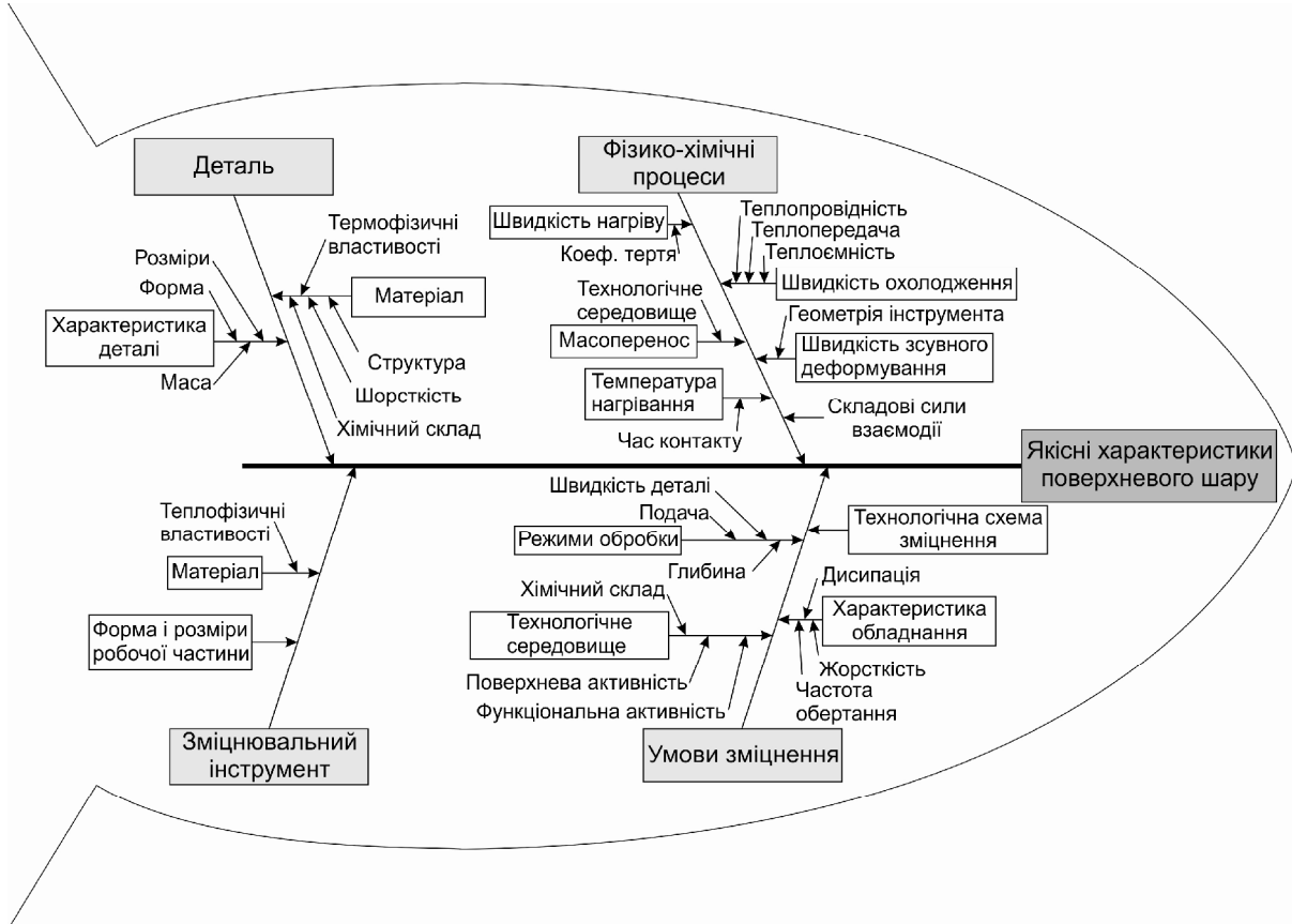
Рис. 2. Діаграма Іскави з основними категоріями причин фрикційного зміцнення деталей машин
