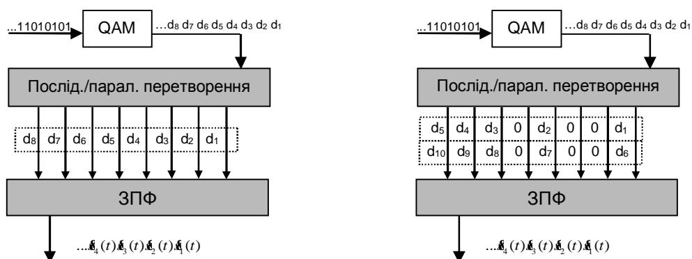
Рис. 2. Схема формування комплексних огинаючих OFDM-символів
