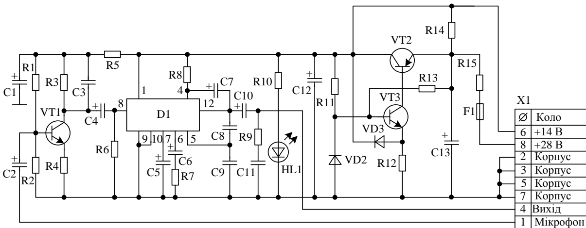
Рис. 4. Схема принципова електрична пристрою
