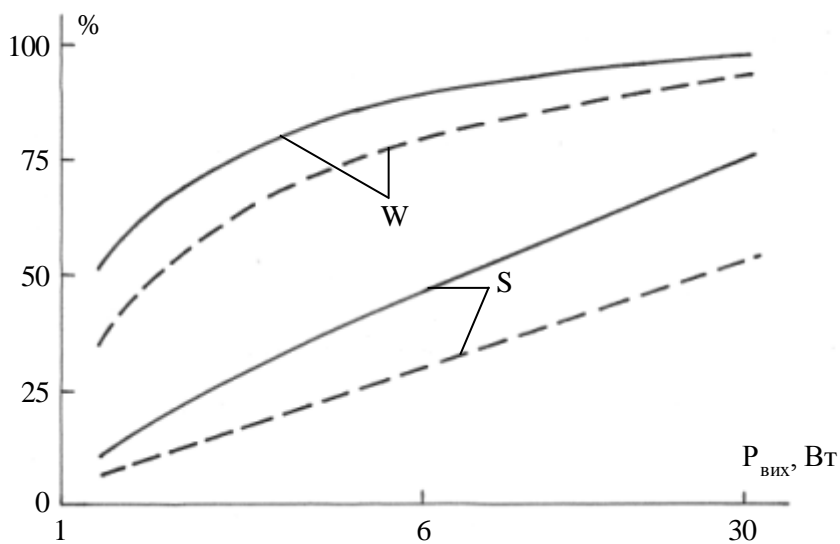
Рис. 2. Залежність складової S та словесної W розбірливостей мовного повідомлення від вихідної потужності ПНЧ: суцільна лінія – для оптимальної АЧХ звукового тракту; пунктирна – для рівномірної АЧХ
