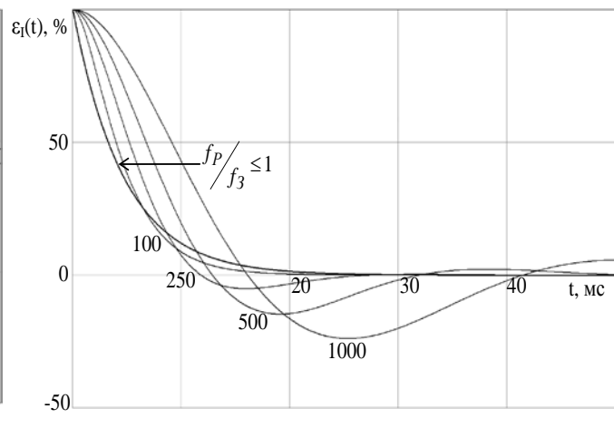
Рис.4. Динамічна похибка встановлення струму в індуктивній складовій комплексного навантаження при зміні смуги пропускання ПНС.
