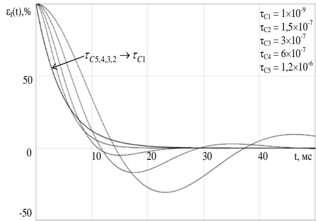
Рис.8. Динамічна похибка встановлення струму в індуктивній складовій комплексного навантаження при різних значеннях ємності навантаження ПНС.
