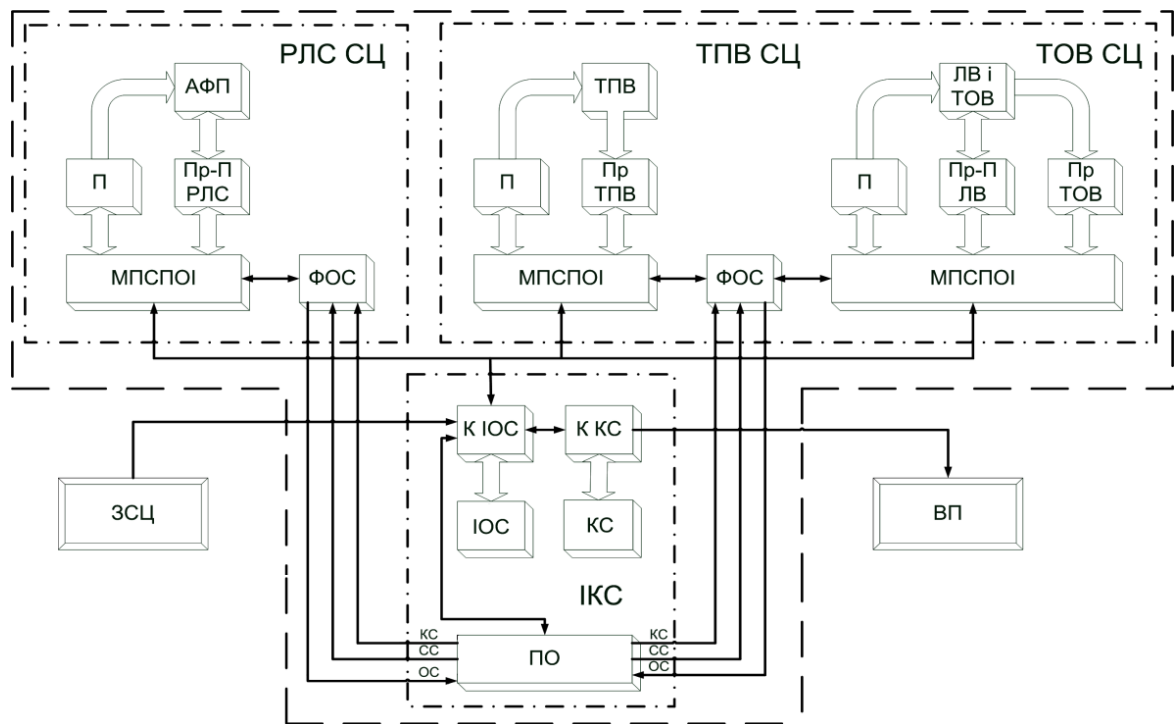
Рис. 1. Структурна схема радіоелектронного комплексу моніторингу повітряного простору.
