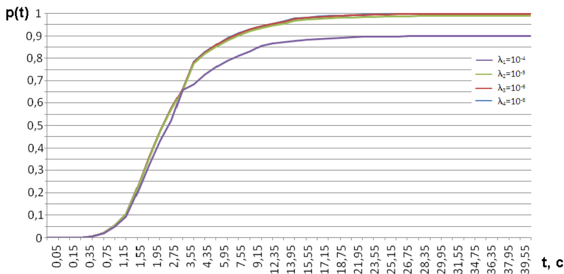
Рис. 3. Графік визначення ймовірності успішного виконання цільової функції РЕК моніторингу повітряного простору при зміні інтенсивностей відмов апаратних засобів.
