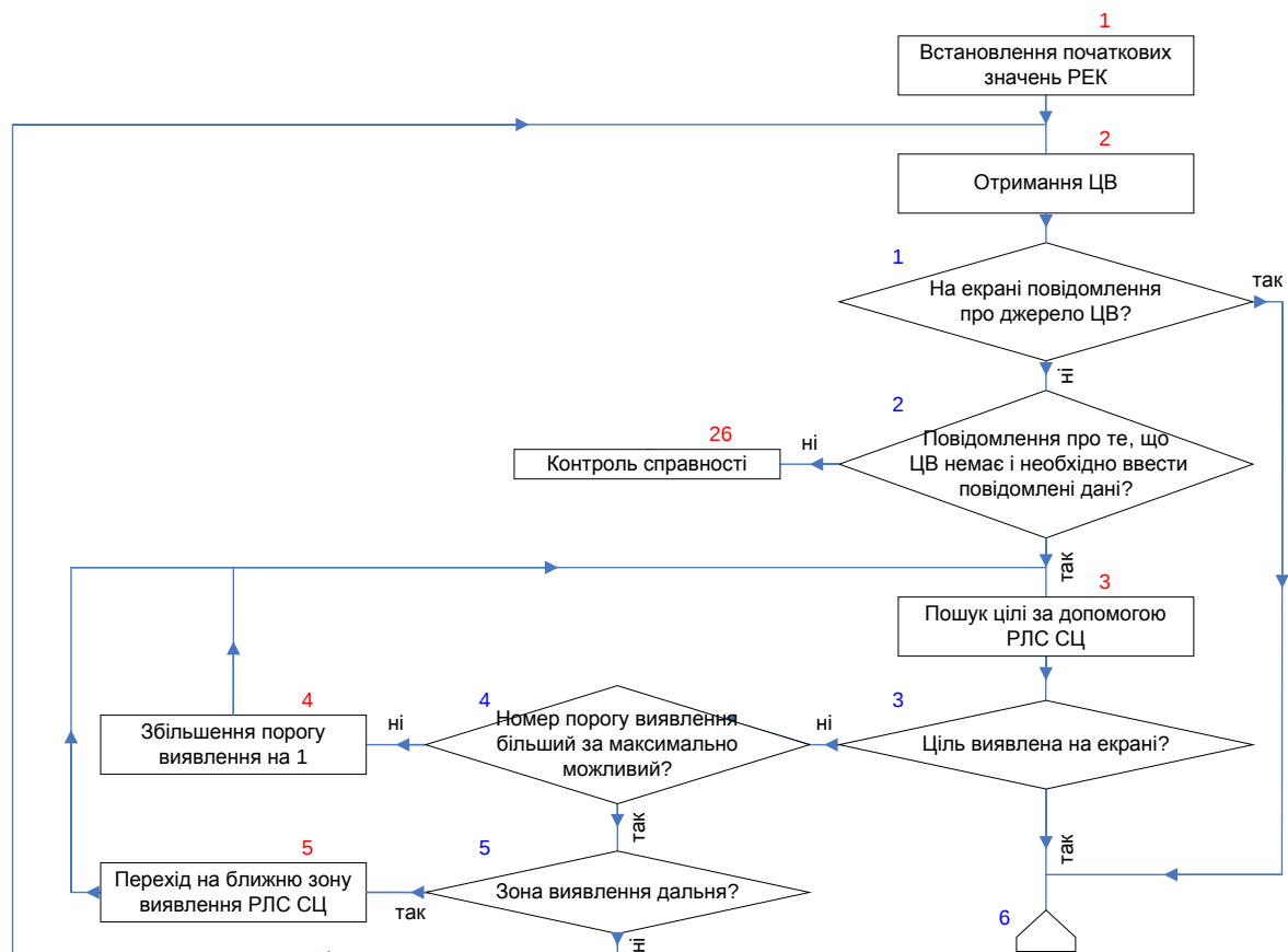
Рис. 2. Фрагмент еквівалентного алгоритму функціональної поведінки РЕК.
