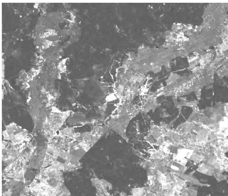
Рис. 4. Вхідне (а) та виправлене (б) зображення Landsat7 (3-й канал)
