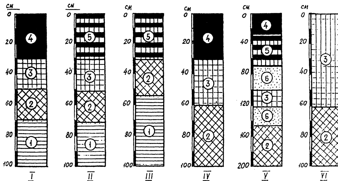
Рис. 1. Моделі генетичної будови техноземів (за Р.М. Панасом, 2005): 1 – токсичні породи; 2 – водонепроникні породи; 3 – потенційно-родючі породи; 4 – родючий ґрунт; 5 – потенційно-родючі породи меліоровані; 6 – пісок
