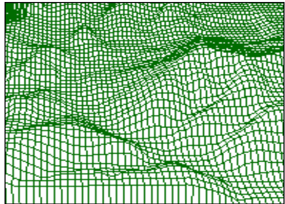
Мал.10. Каркасна ЦМР на район Східниці, утворена регулярною сіткою планово-висотних точок.
