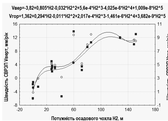
Рис. 2. Лінійна та поліноміальна апроксимації швидкостей СВРЗП (що визначені по вертикальному V верт та горизонтальному V гор розчленуванням рельєфу) і а) відміток поверхні кристалічного фундаменту; б) відміток денної поверхні; в) потужності осадового чохла
