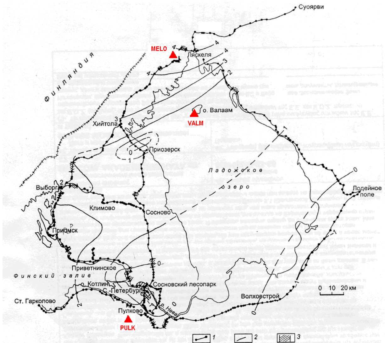
Рис. 2. Схема нивелирной сети и карта современных вертикальных движений земной поверхности Карельского перешейка: 1 — нивелирные линии и репера, 2 — изолинии скоростей и мм/год, 3 — зоны контрастных движений (Энман, 2006). Красными треугольниками показаны GPS пункты
