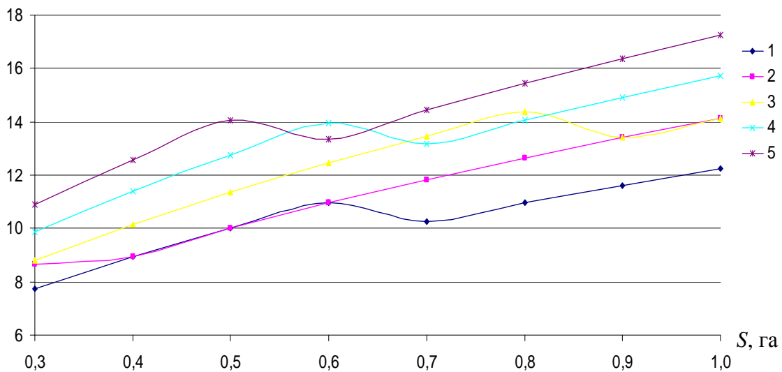
Рис. 3. Графік залежності середніх квадратичних похибок площ земельних ділянок від 0,30 га до 1,0 га від коефіцієнта видовженості при t_{x,y} згідно з [6]
