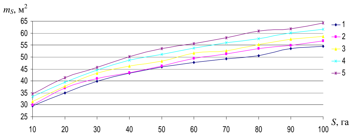
Рис. 5. Графік залежності середніх квадратичних похибок площ земельних ділянок від 10 га до 100 га від коефіцієнта видовженості при t_{x,y} згідно з [6]
