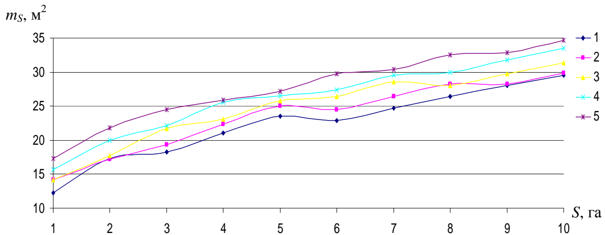
Рис. 4. Графік залежності середніх квадратичних похибок площ земельних ділянок від 1 га до 10 га від коефіцієнта видовженості при t_{x,y} згідно з [6]
