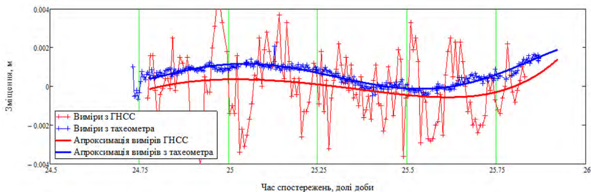
Рис. 10. Зміщення референційної ГНСС-станції BRGN по осі Y (Схід-Захід) за результатами лінійно-кутових та супутникових вимірювань
