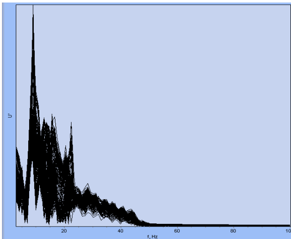
Рис. 6а. Спектр x компоненти швидкості переміщення Fig. 6a. The range of x velocity components
