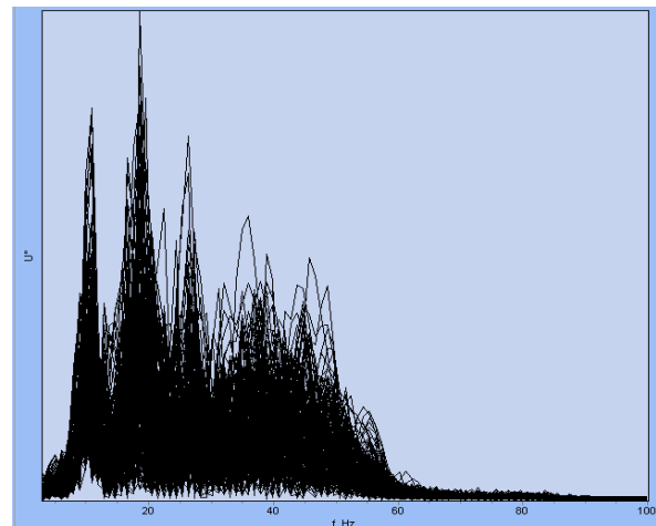
Рис. 7б. Спектр y компоненти прискорення Fig. 7b. The range of y acceleration components
