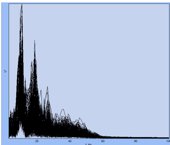
Рис. 6б. Спектр y компоненти швидкості переміщення Fig. 6b. The range of y velocity components
