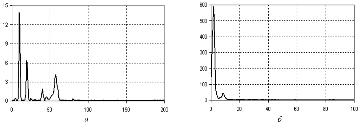
Рис. 7. Графік спектральної густини вібраційного сигналу від сівалки: а – з затисненими болтами; б – з послабленими болтами
