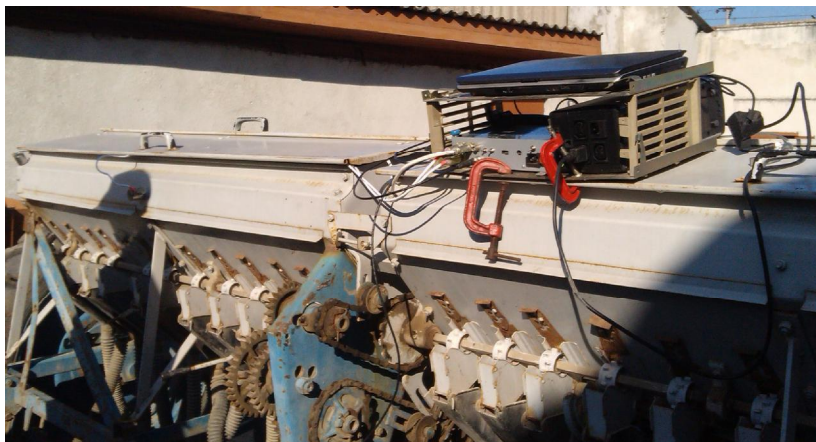
Рис. 4. Розташування комплексу віброметрії на сівалці
