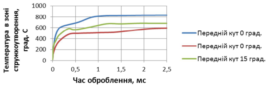
Рис. 14. Графіки залежності температурних показників різання від геометрії різального інструменту
