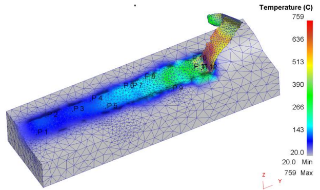
Рис. 3. Результати реологічного моделювання зони концентрації теплового поля на передній поверхні різця (а) та вздовж обробленої поверхні заготовки (б) (інструмент умовно не показаний) у системі Deform 3D
