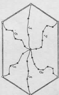
Рис. 5. Проект полигонометрической сети.
