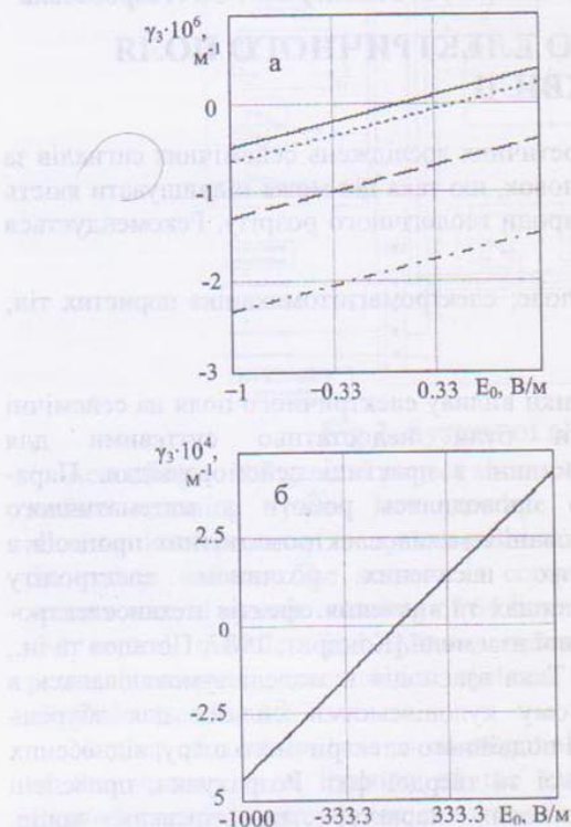
Рис. 1 Залежність коефіцієнта загасання хвилі першого роду від величини і напрямку слабого (а) і сильного (б) зовнішнього електричного поля для частот \omega=100, 200, 400, 600 \text{ c}^{-1} (суцільні, пунктирні, штрихові і штрих-пунктирні лінії) за \gamma_{\sigma} = 3 \cdot 10^{-8} \text{ Па}^{-1}
