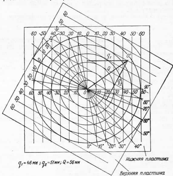
Рис. 2. Палетка для определения полного крена сооружения.
