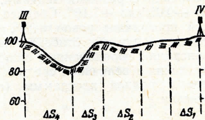
Схема профиля по направлению III—IV.
