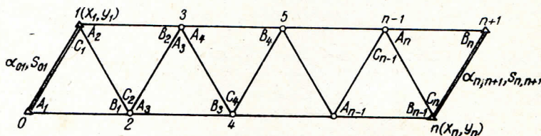
Рис. 1. Схема цепи треугольников.
