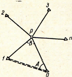
Рис. 4. Схема многолучевой линейной засечки.
