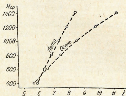
Рис. 2. График зависимости времени утреннего максимума рефракции от средней высоты луча.
