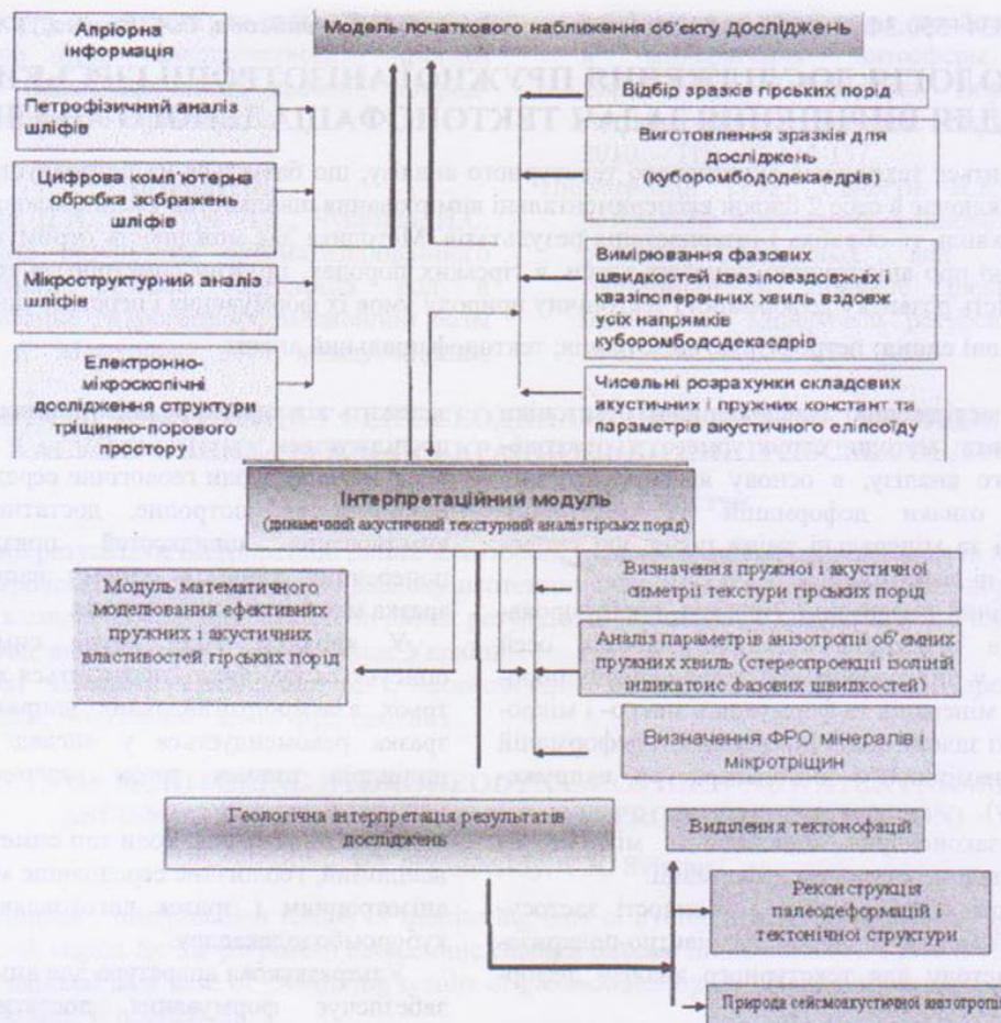
Рис. 1 Схема вимірювально-інтерпретаційної технології
