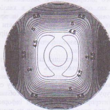
Рис. 3. Стереопроєкція вказівної поверхні фазової швидкості квазіповздожньої хвилі біотитового сланцю Криворіжжя
